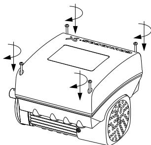
Рис. 61 Установка крышки клеммной коробки
