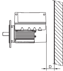
Նկար 1 Նվազագույն հեռավորությունը (D) Էլեկտրական շարժիչի միջև պատը կամ այլ անշարժ օբյեկտները
