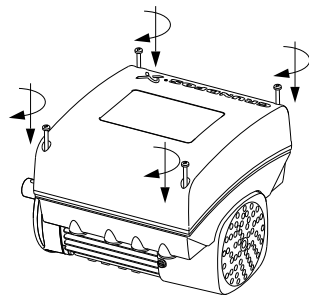
61-сурет Клеммалық қорап қақпағын орнату
