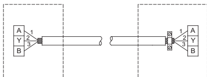
Сүрөт 11 3 жылкалуу экрандаштырылган кабелди туташтыруу
