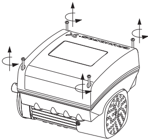
56-сурет Бұрандаларды босату
