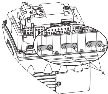
67-сурет Кабельдердің экрандалған орамдарын жерге тұйықтау
