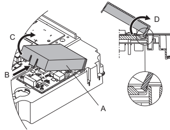
Рис. 64 Снятие крышки модуля СИМ
