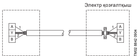
12-сурет 2 тарамды қоршалған кабельді қосу
