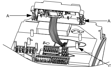
60-сурет Пластик қақпақты орналастыру
