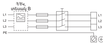
Նկար 6 Էլեկտրասնուցման անջատիչով, ապահովիչներով և լրացուցիչ պաշտպանությամբ ապահովված էլեկտրական շարժիչը ցանցին միանալու օրինակ
