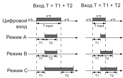
Рис. 42 Функция таймера длительности для цифровых входов
