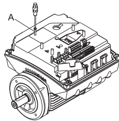
Рис. 65 Снятие крепёжного винта
