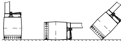
Рис. 5 Размещение Unilift KP-A и Unilift KP-M
