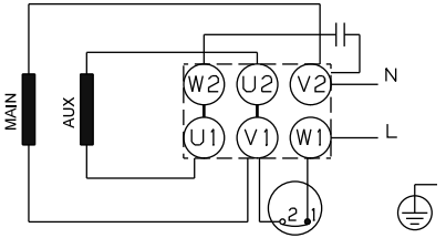
Рис. 14 З'єднання, 220-230 В, 1,1-2,2 кВт
