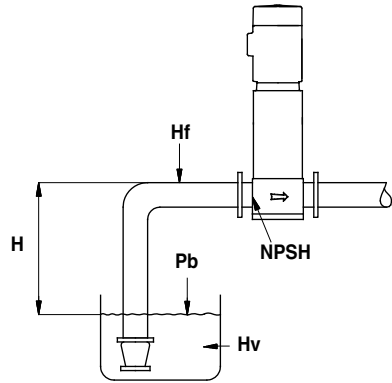
Рис. 21 Схематичне зображення відкритої системи з насосом CR
