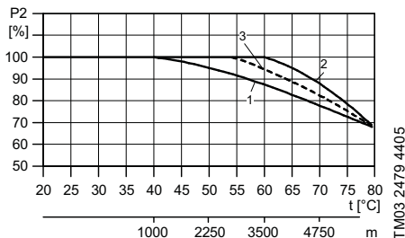
Рис. 19 Вихідна потужність двигуна в залежності від температури та висоти
