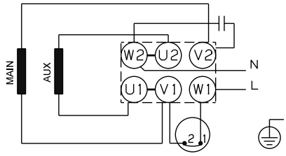
Рис. 15 З'єднання, 240 В, 1,1-2,2 кВт
