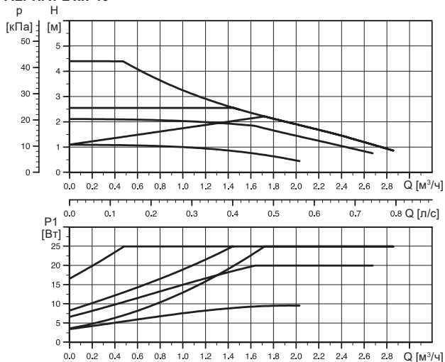
Рис. 16 Расходно-напорная характеристика насосов серии ALPHA1 L
